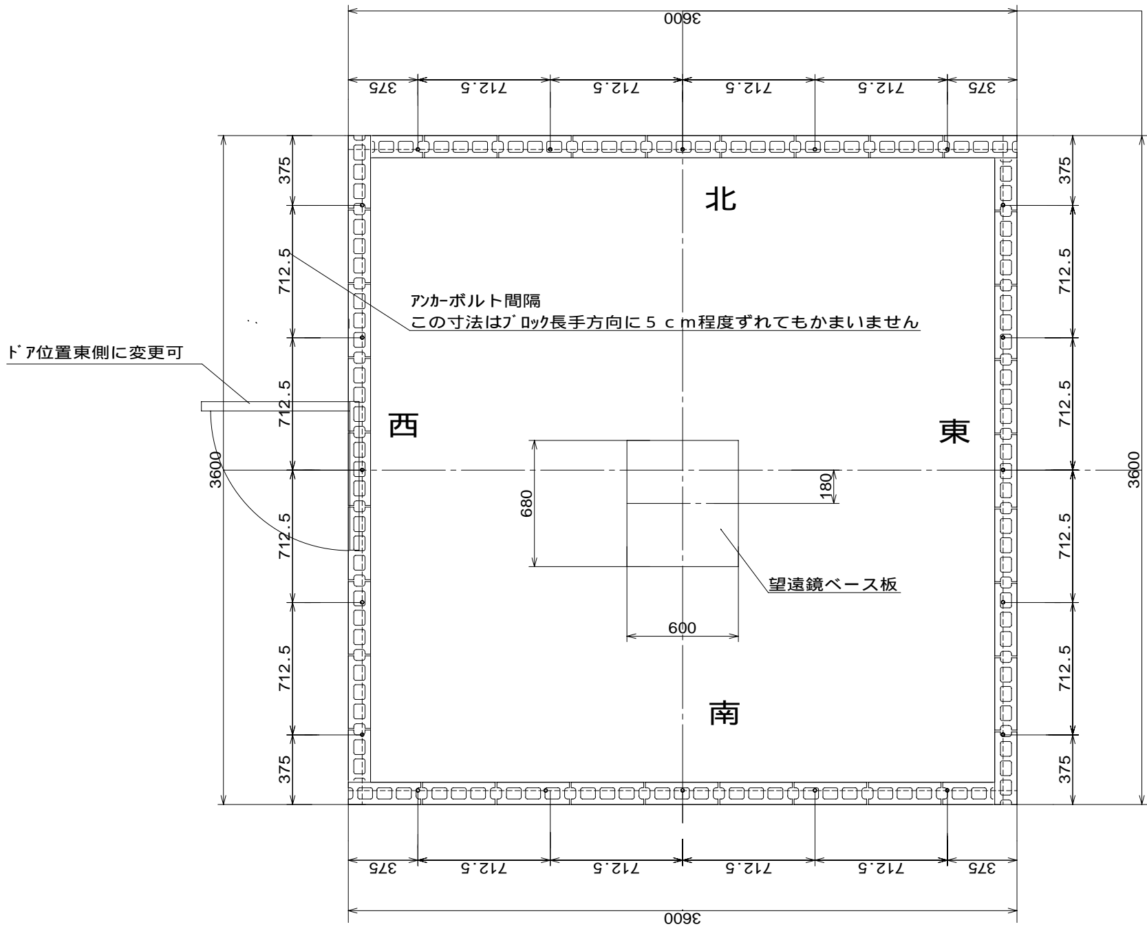
スライドルフスーパー3636基礎参考図
