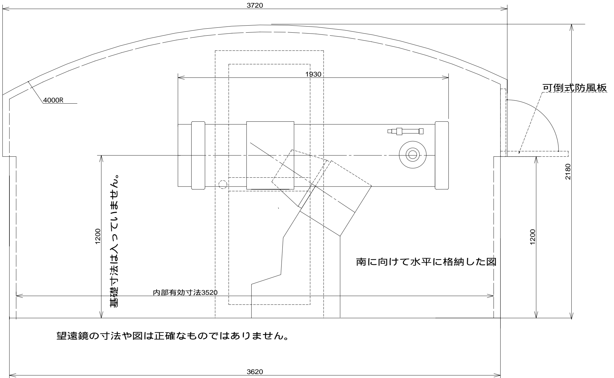
スライドルーフ3600×3600に入れた40cmニュートン式反射望遠鏡を格納した状態の予想図
