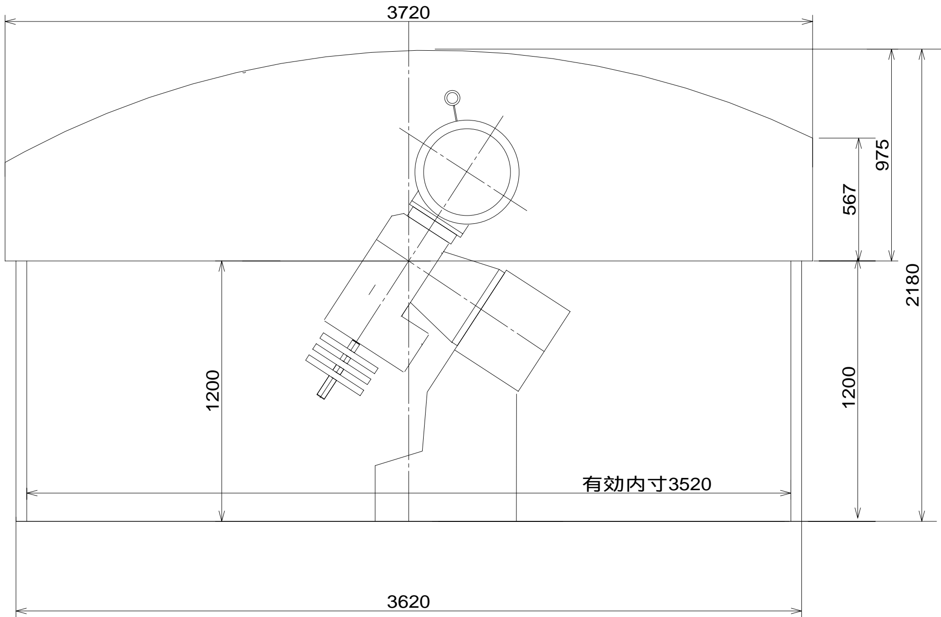
スライドラーフ3600 × 3600に入れた40cmニュートン式反射望遠鏡を東西方向に格納した状態の予想図
